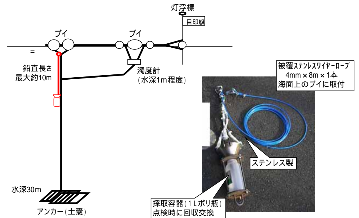
（簡易セジメントトラップ設置状況概要図）
