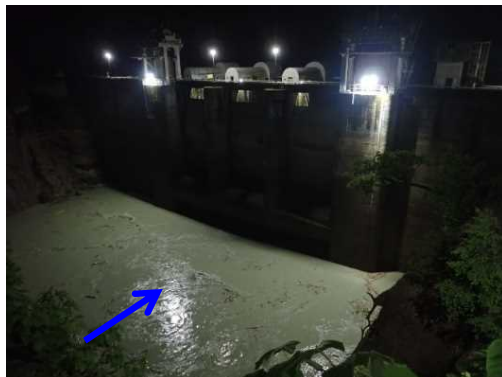
【出し平ダム排砂路呑口部】水位低下中 (EL. 315.88m) 7月1日 22:40撮影
