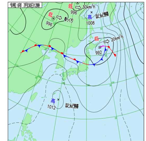
天気図(7月30日12時)
