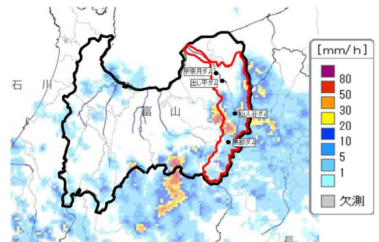
レーダ雨量(7月30日 15時30分)
