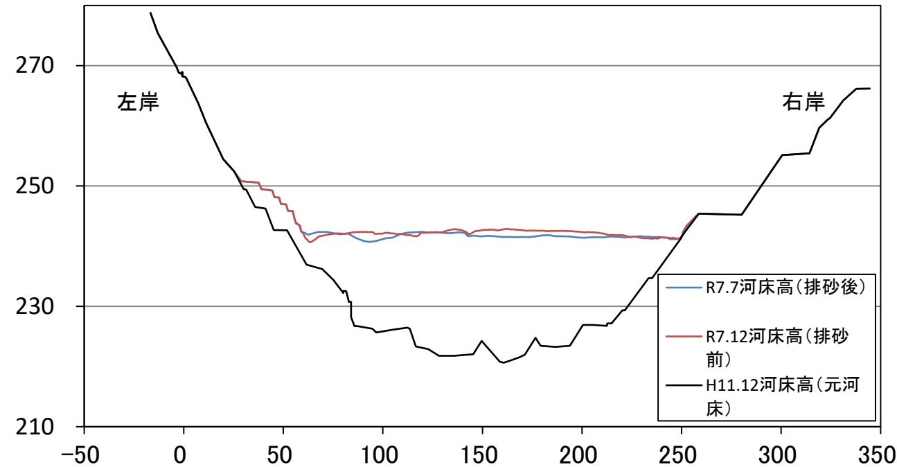
22.6k横断面図
