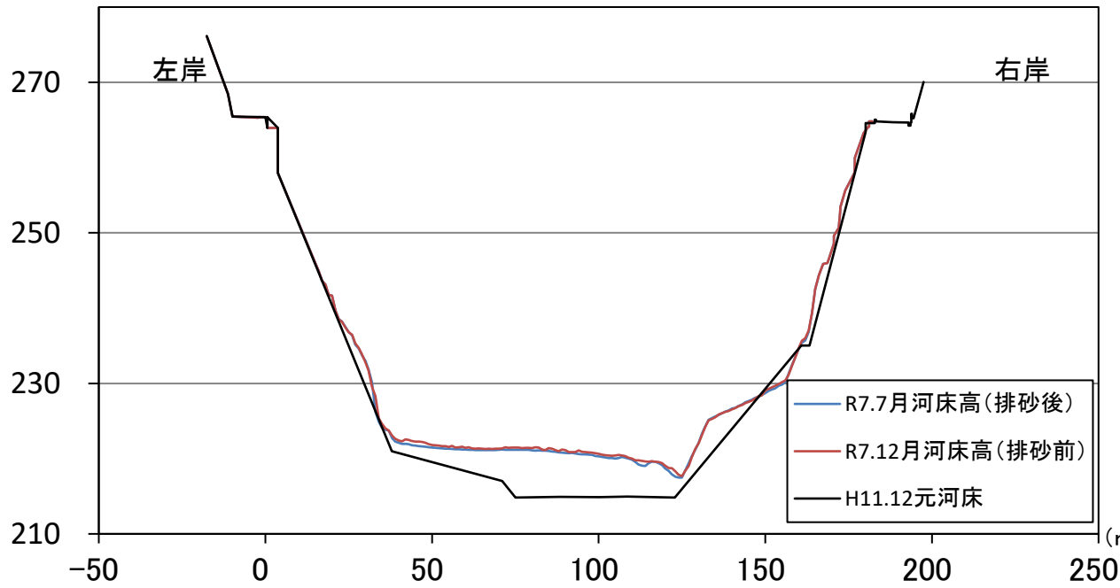
20.8k横断面図
