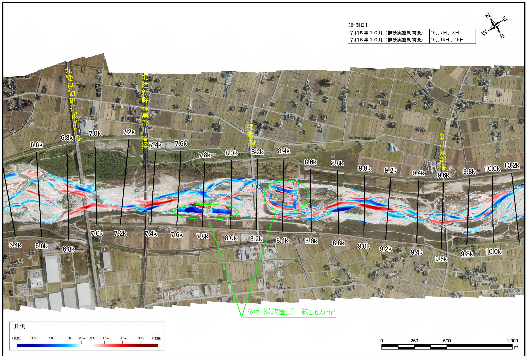
黒部川(3)標高差分図(令和6年10月－令和5年10月)
