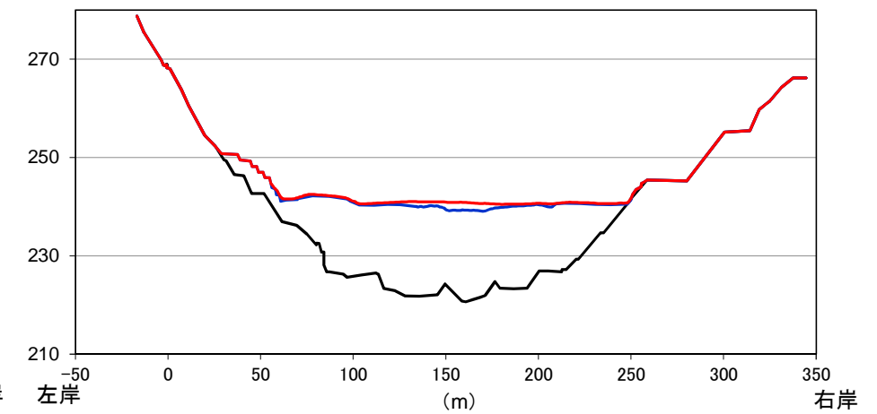
22.6k横断面図
