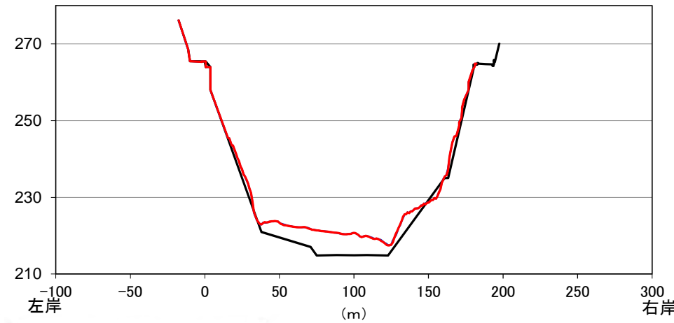
20.8k横断面図
