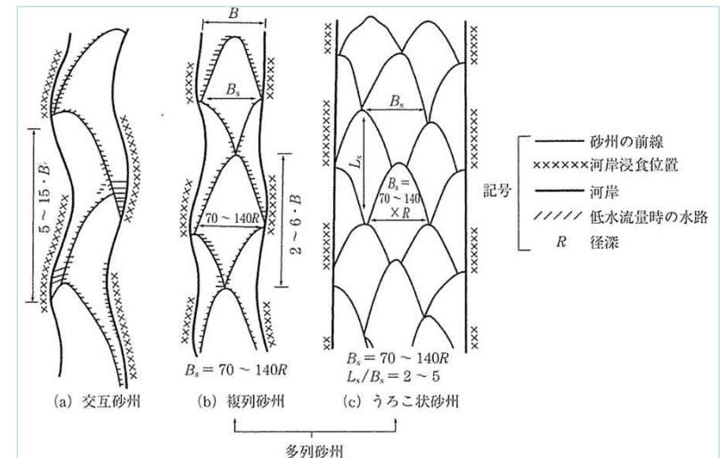
図 10.1 典型的な砂州のスケール
