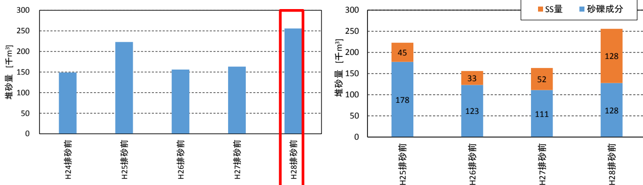
図1. 排砂前※までの宇奈月ダム堆砂量とシミュレーションによる堆砂量内訳
