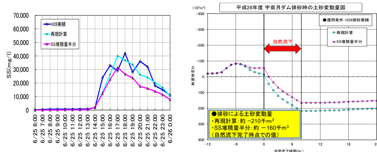
図3. SS堆積量を半にした条件での放流SS及び土砂変動量図
