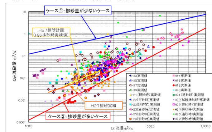
【出し平ダムにおける流量と流砂量の関係】
