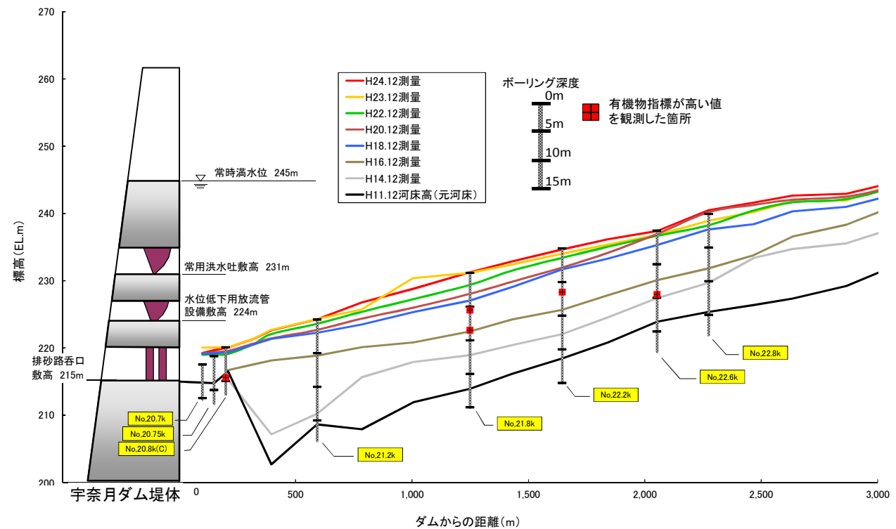
図 宇奈月ダム貯水池縦断面図と有機物指標が高い値を観測した箇所の位置図
