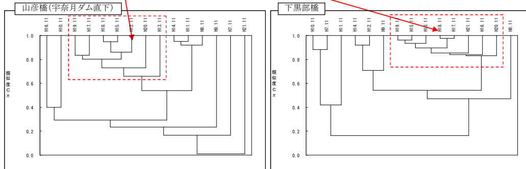
図3-3-6 類似度(秋季)
