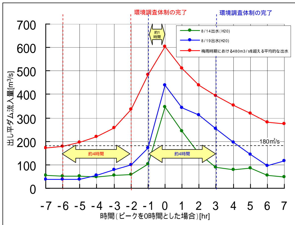
図2 短時間集中豪雨の例(出し平ダム)
