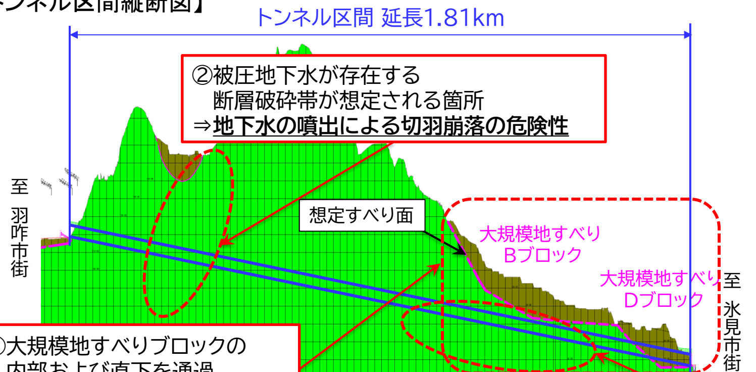
【トンネル区間縦断図】
