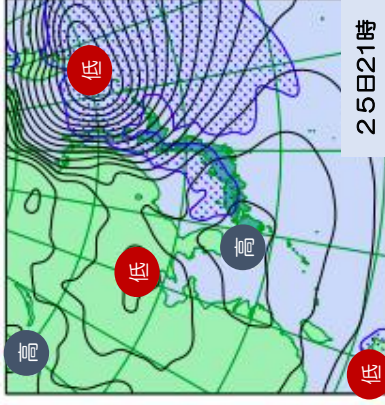
陰影域：24時間降水量予想が5ミリ以上の範囲
