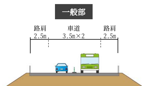
標準横断図（暫定2車線）
