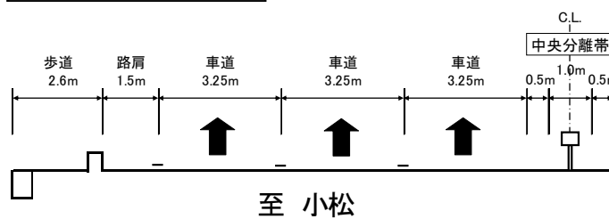
整備後 (3車線)
