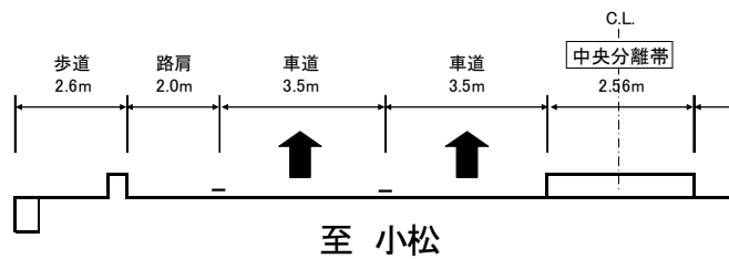
整備前 (2車線)
