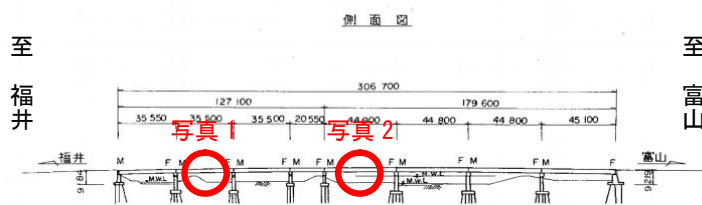
【犀川橋(下り)一般図】
