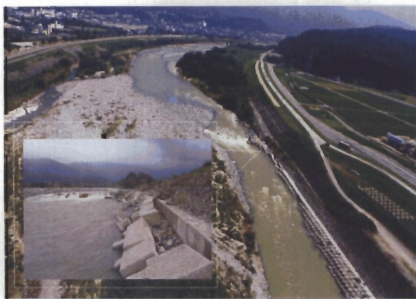
手取川被災箇所（根固工流出） 石川県能美市灯台橋地先
