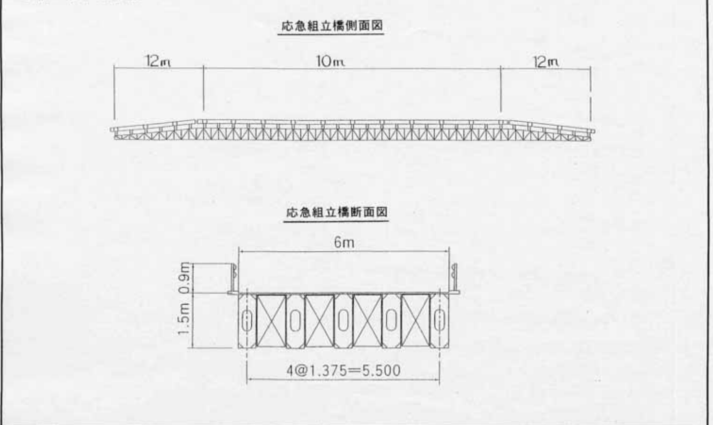
応急復旧標準断面図
