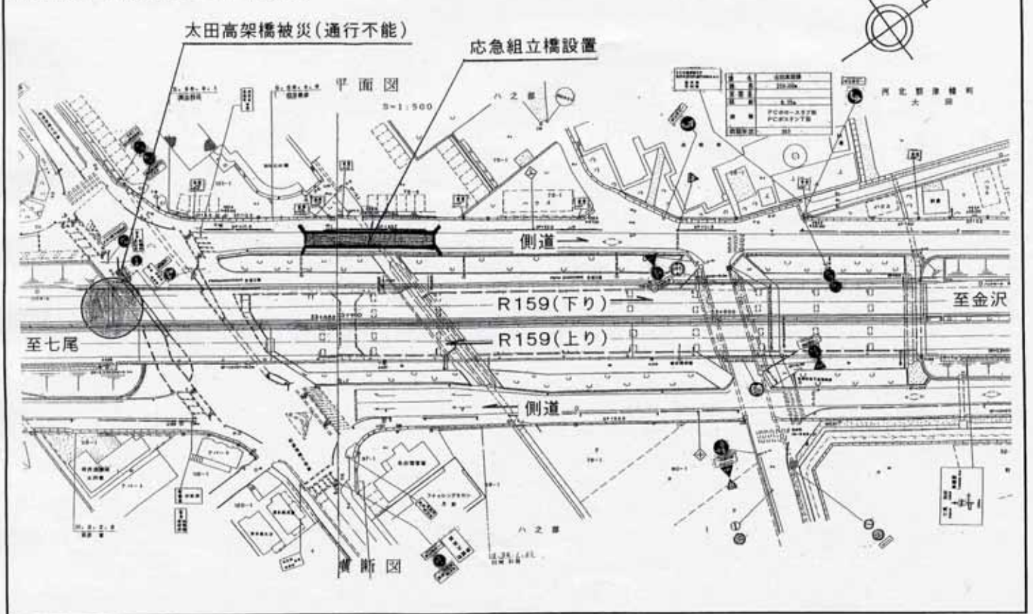
応急復旧平面図(S=1:1000)
