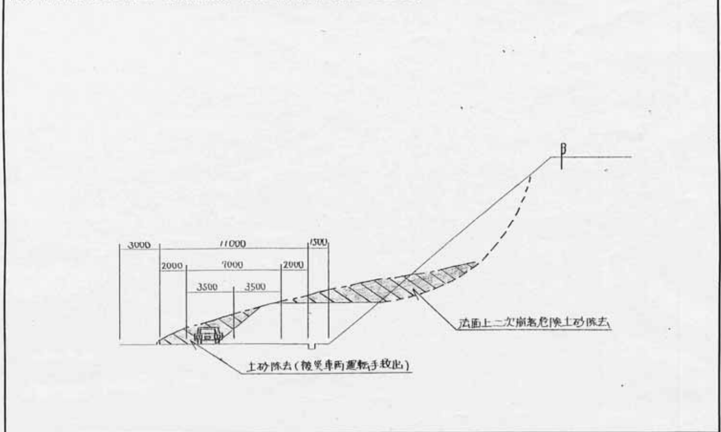
被災車両救出及び法面上二次崩落危険土砂除去標準断面図(S=1:200)
