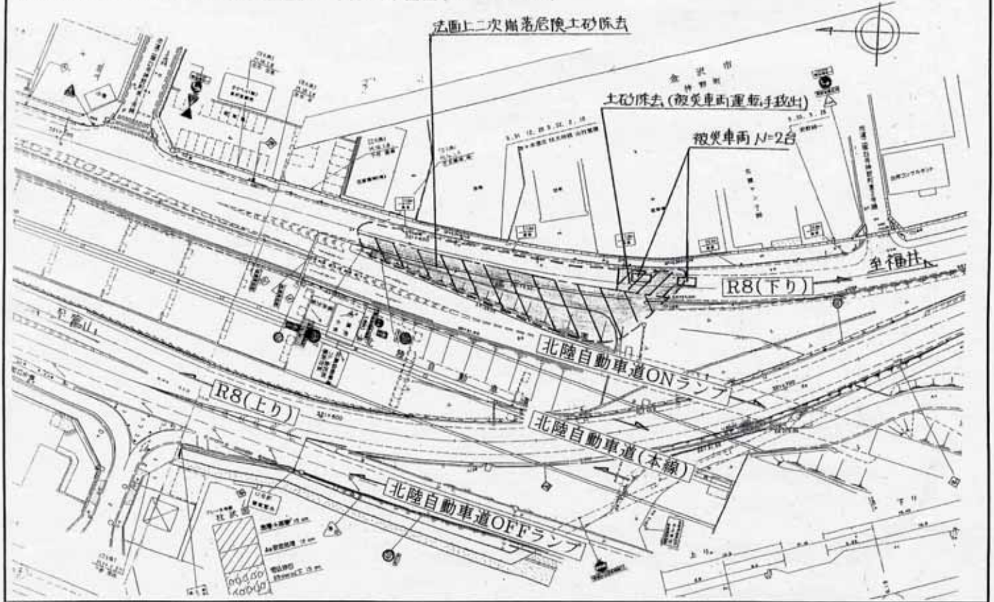
被災車両救出及び法面上二次崩落危険土砂除去平面図(S=1:1000)
