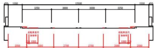
【浅野川大橋 歩道拡幅工事 イメージ図】
