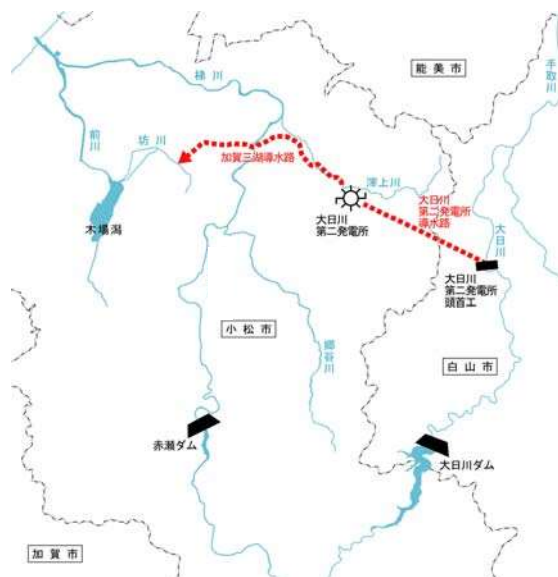
図 6-3 加賀三湖導水路図
