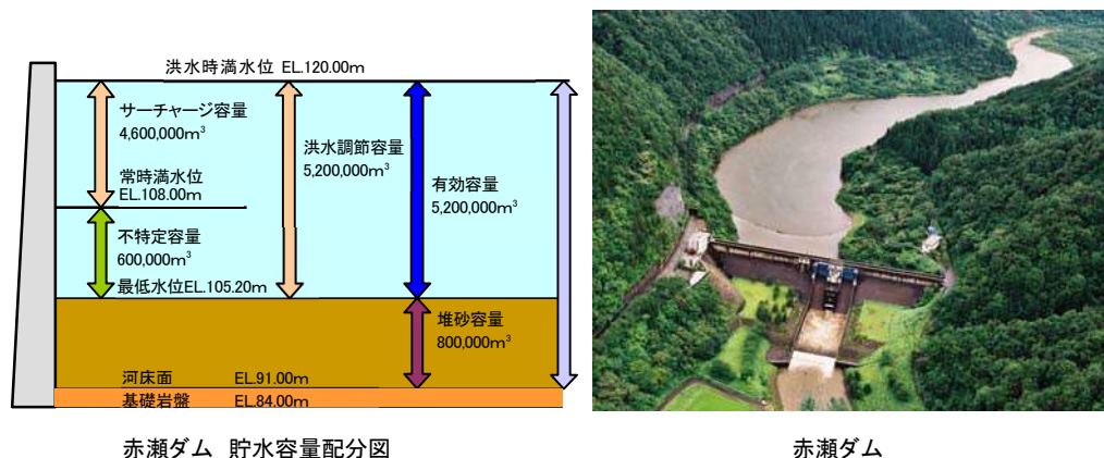
図 3-1 赤瀬ダムの概要
