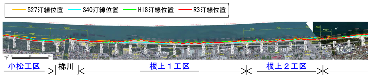
図 5-1 梯川周辺の汀線変化状況
