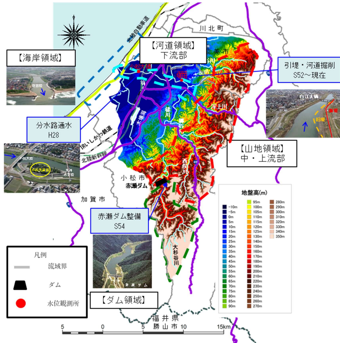
図 1-2 梯川水系流域地形図
