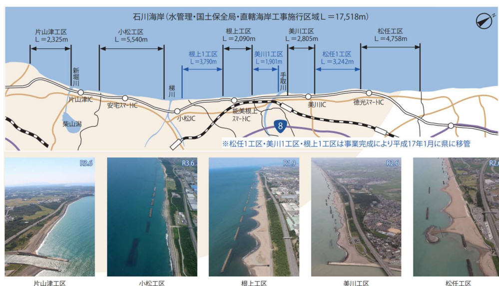
図 5-2 石川海岸の施工区域
