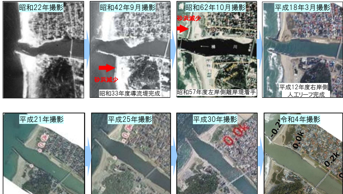
図 4-5 河口部平面形状の変化
