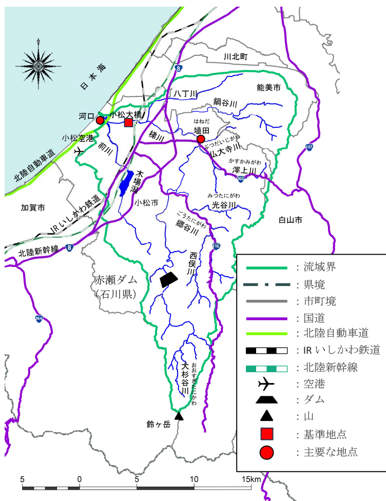
図 1-1 梯川流域図
