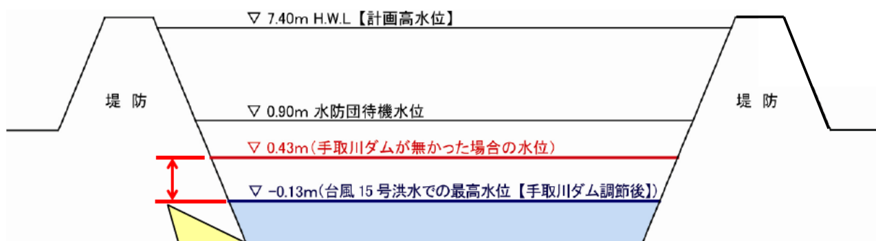
【河川横断面図(鶴来地点)】
