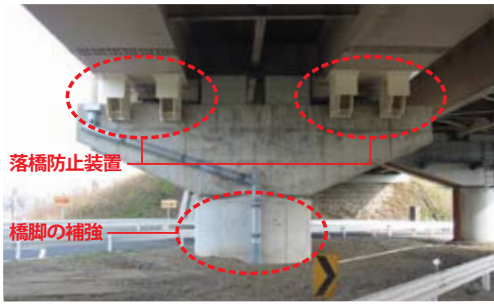
補強後/地震による甚大な被害を防ぐため、落橋防止装置の設置や、橋脚の補強を実施
