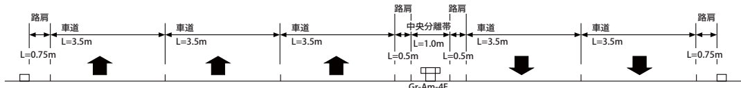
● 5車線化道路断面図【一般部】(総幅員 21.0m)
