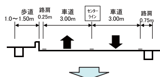
● 歩道計画断面図【一般部】(総幅員 13.0m)
