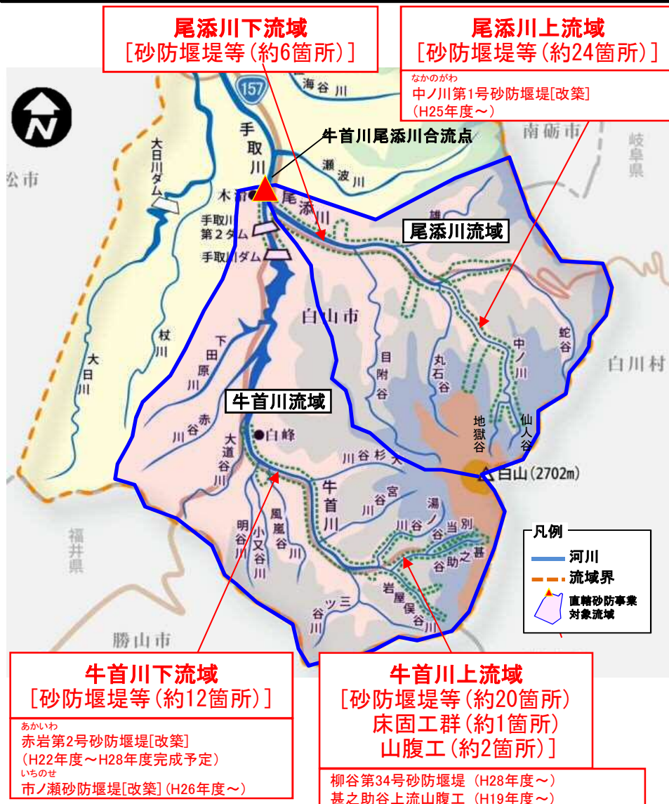
図3-1 中期的な目標の計画箇所
