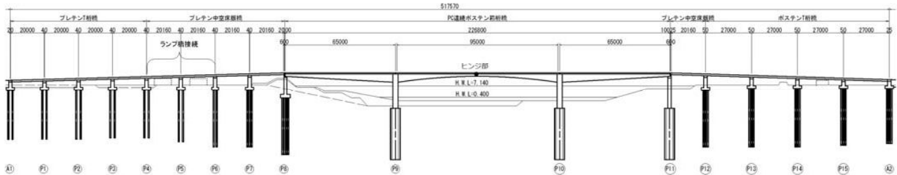
断面図
