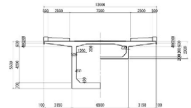
断面図
