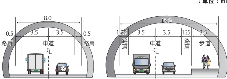
【標準断面図(トンネル部)】
