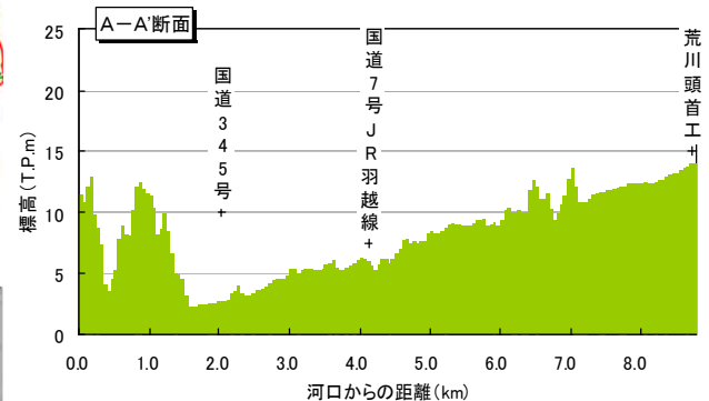
荒川流域断面図(写真 A-A' 断面)
