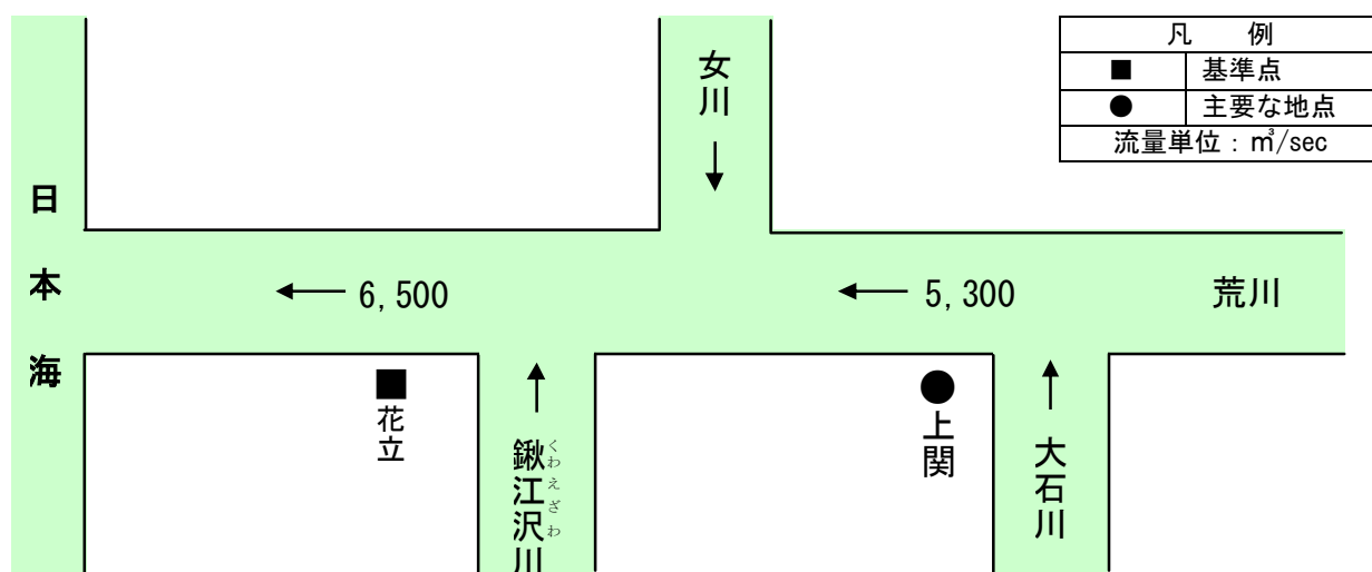
荒川計画高水流量図
