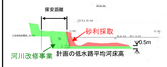
貝附地区河道掘削 標準断面図
