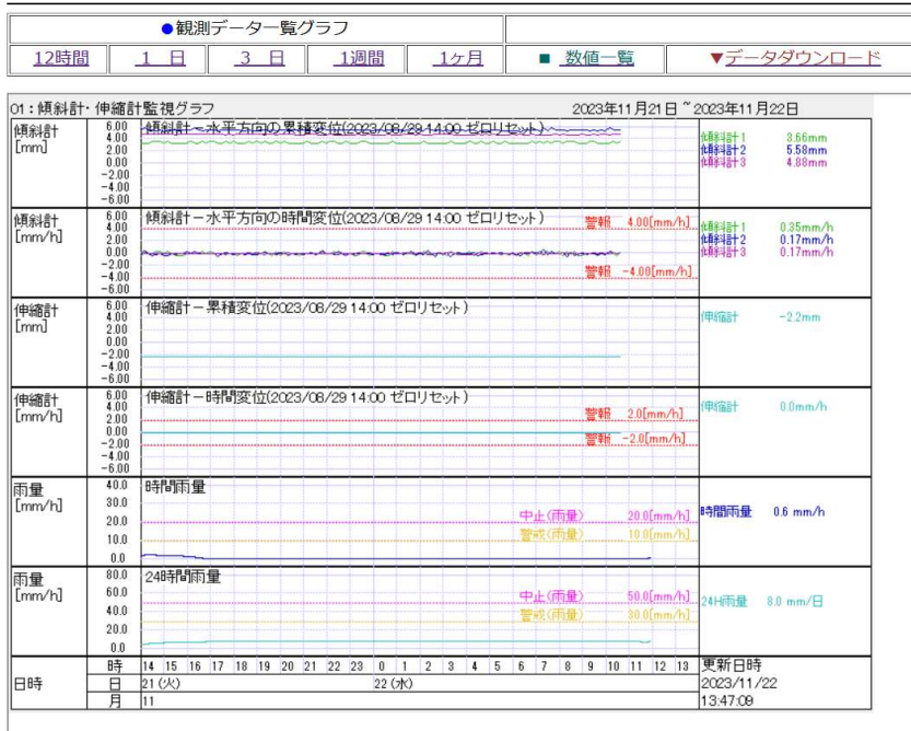
令和5年度右保谷第4号砂防堰堤林道付替工事 傾斜監視システム 美笠建設株式会社
