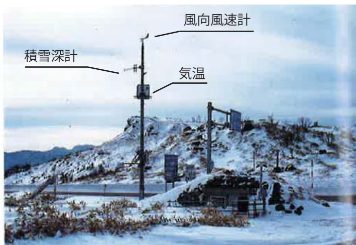
②気象観測センサー
