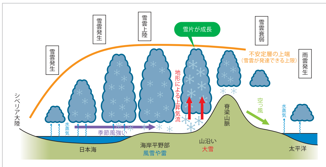
①山雪の概念図
