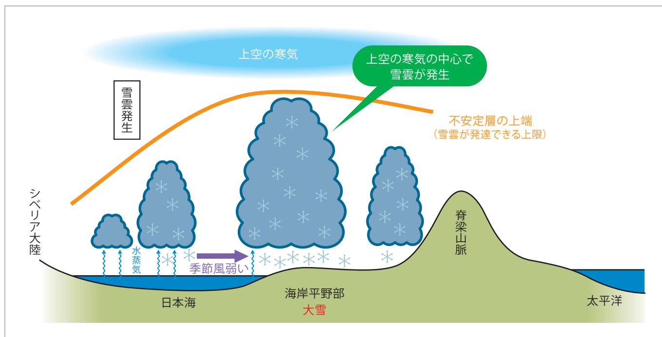
②里雪の概念図
