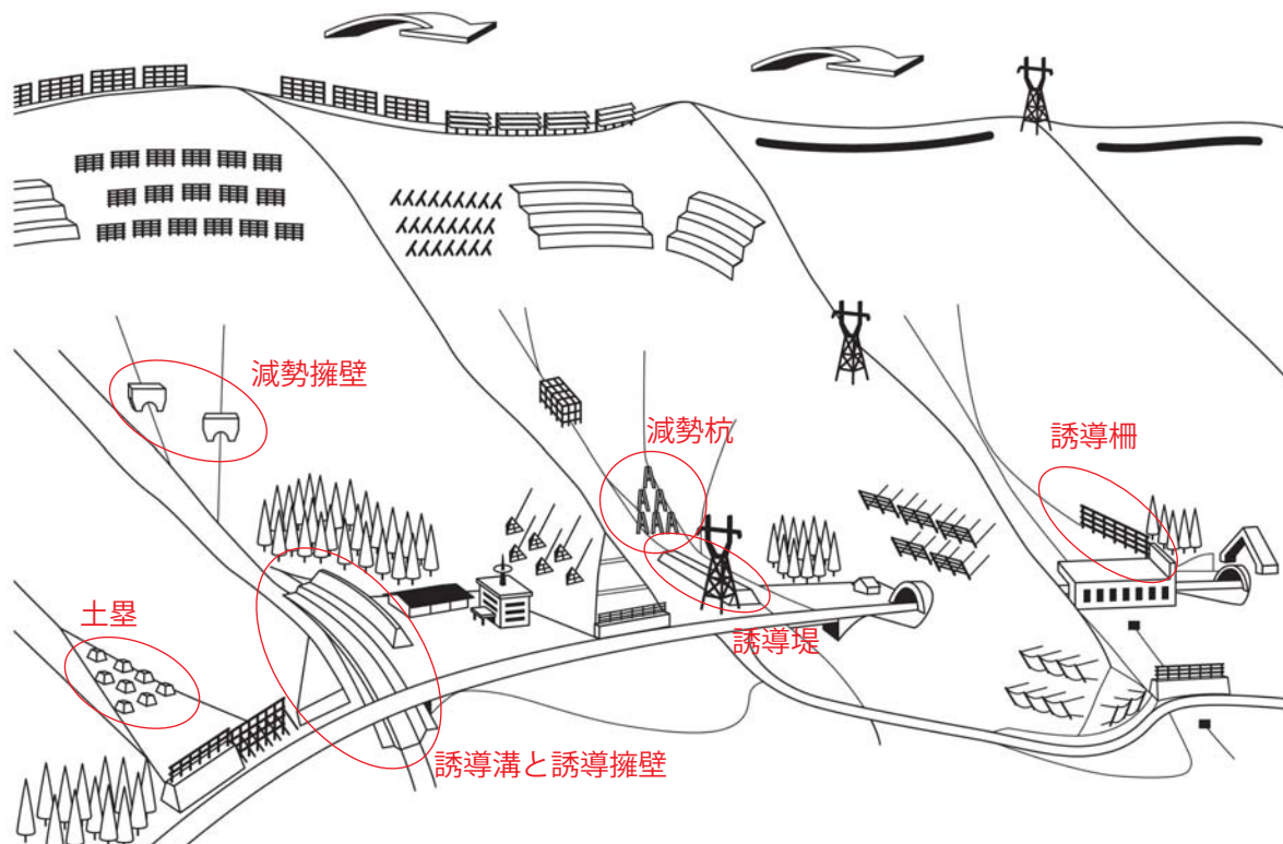
③減勢工と誘導工の役割
