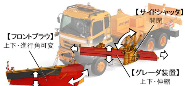
図-1 除雪トラック作業装置
