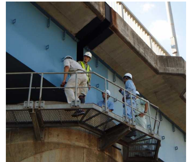
検査路での近接目視点検 (新潟県 三条大橋)
