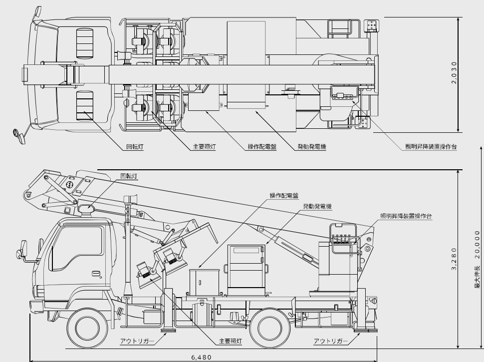
車両外形図
