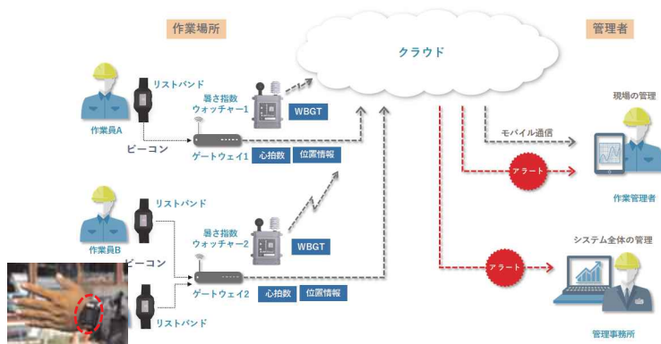
体調管理システムの活用 バイタルセンサーにより心拍数を管理し、複数箇所計測したWBGT値を紐づけ、特定の閾値を一定時間超えた場合にアラートメールを発信
