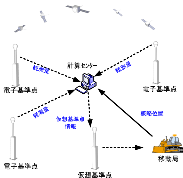
図 2.7 ネットワーク型R T K－G N S S（V R S方式）
