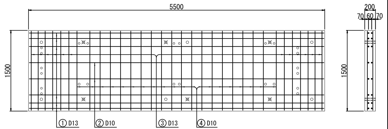
配 筋 図 (参考)
