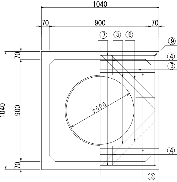
下部平面図
