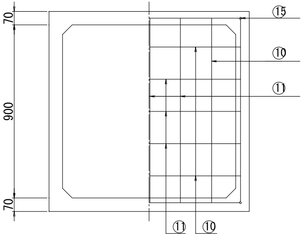
下部平面図
