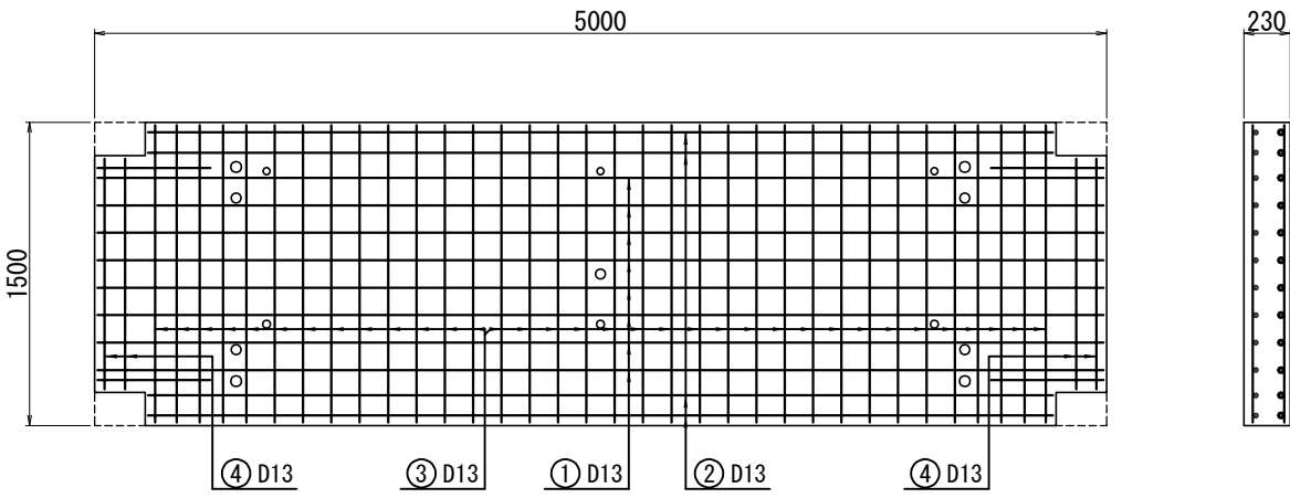
配筋図（参考）
