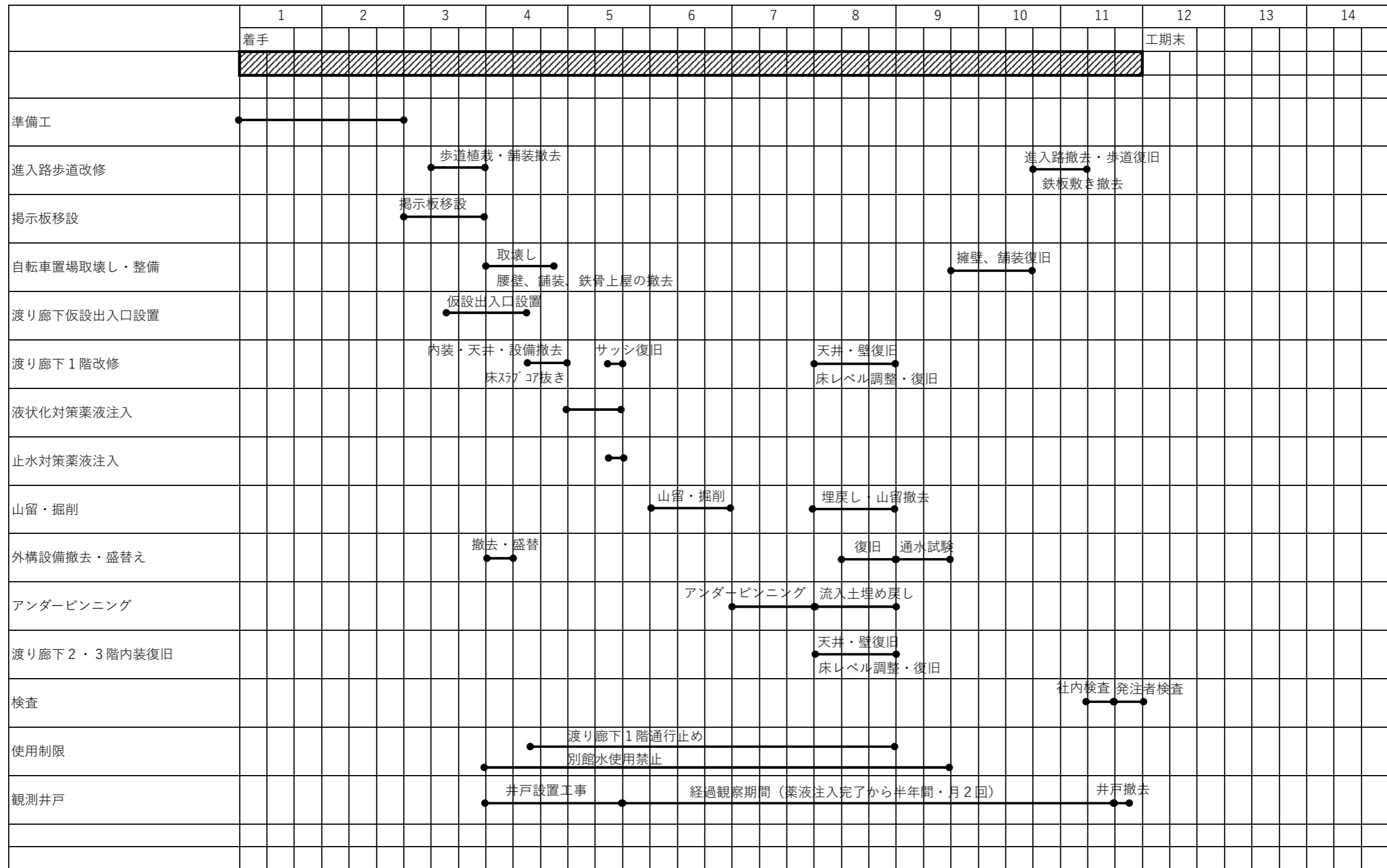
金沢駅西合同庁舎（26）渡り廊下その他復旧工事 概略工事工程表
