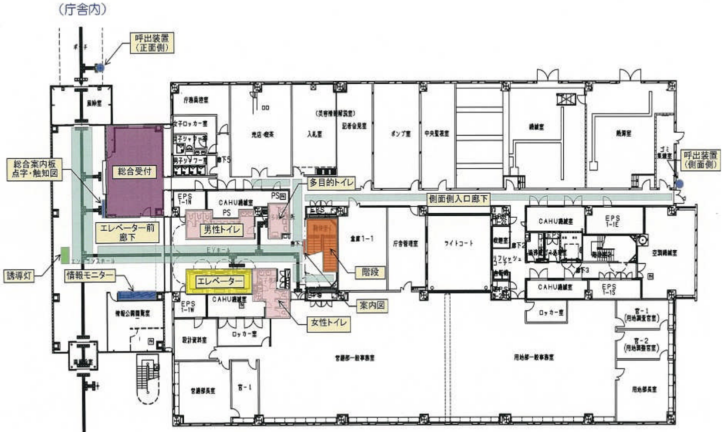
<1階平面図>
