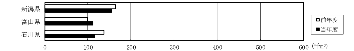
生コンクリート出荷量の推移（１月～３月期）
