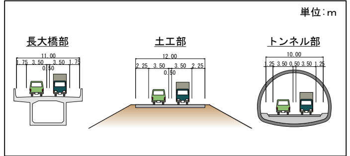
《横断図》
