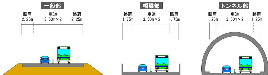
標準横断面図(2車線)
