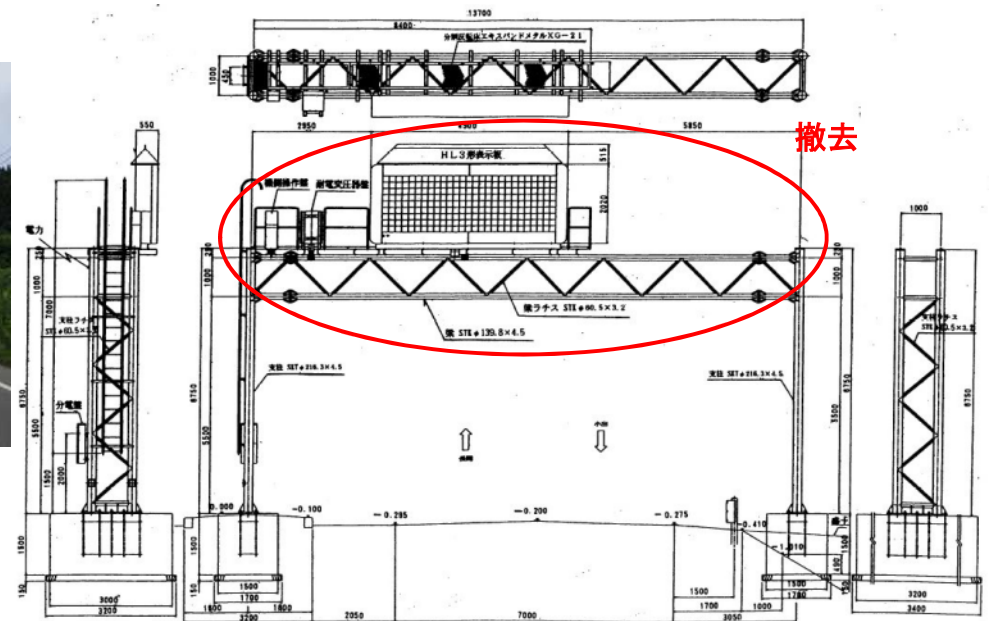
道路情報板立面図
