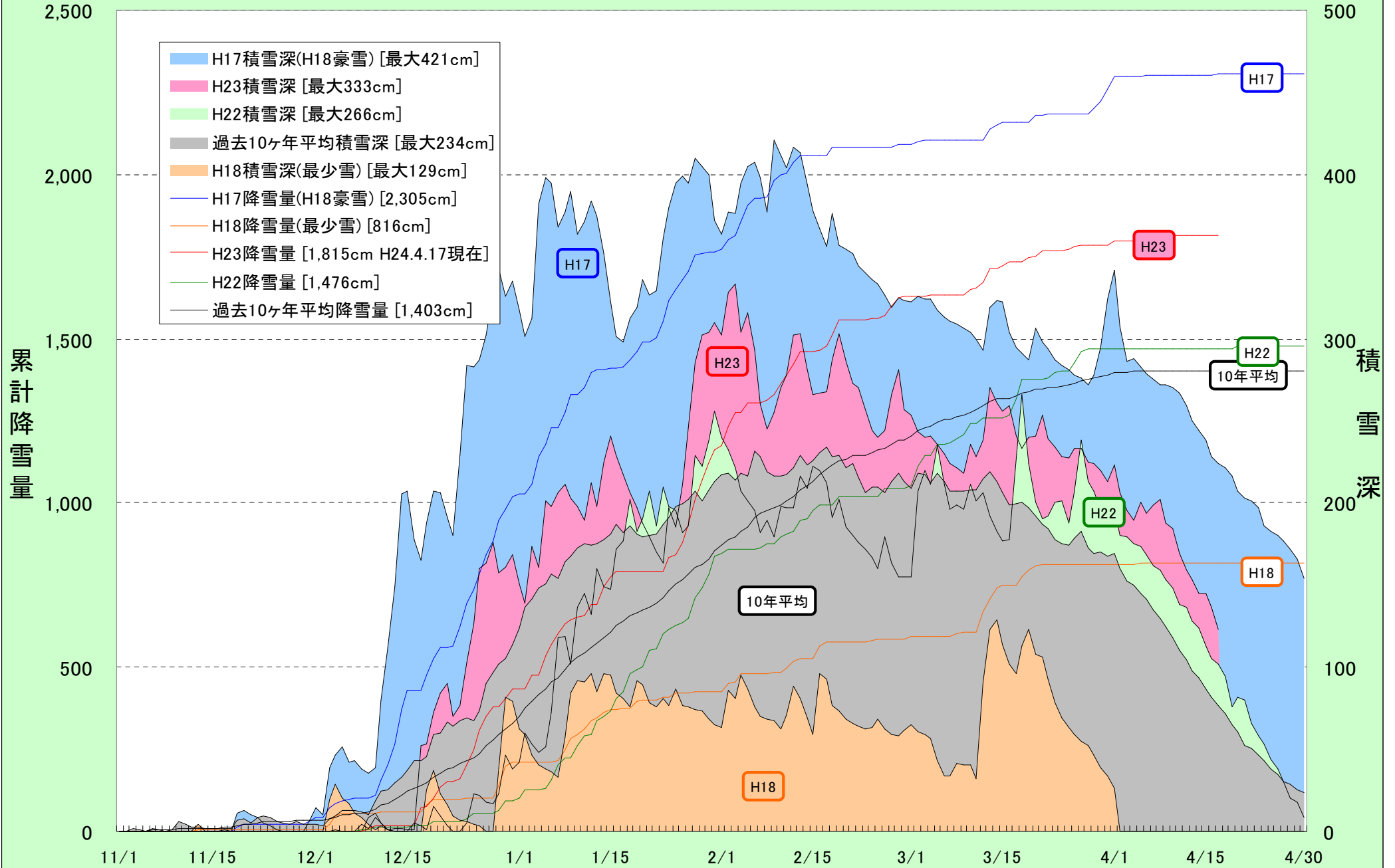
累計降雪量と積雪深の比較（三俣）
