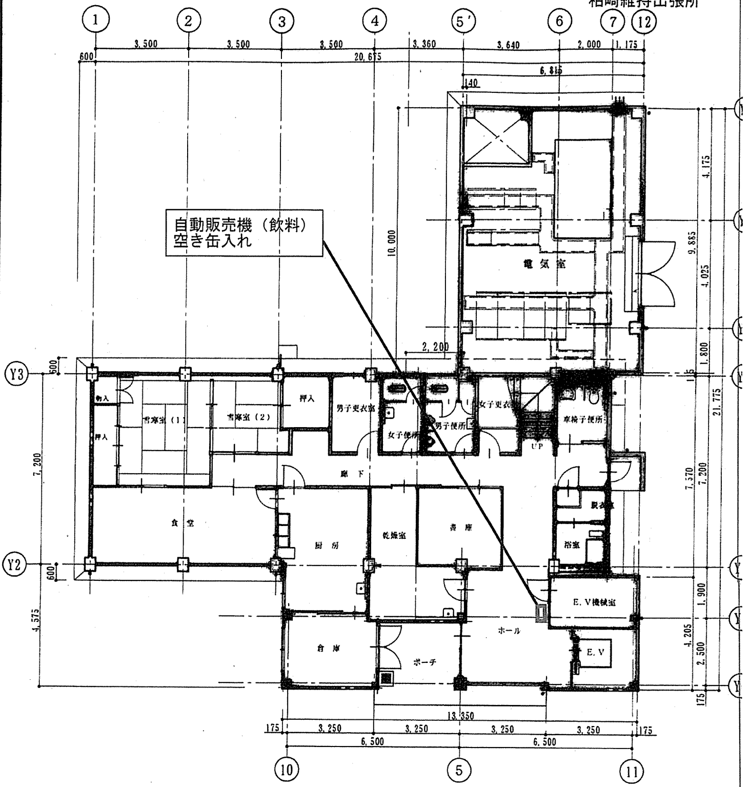
1階平面図
