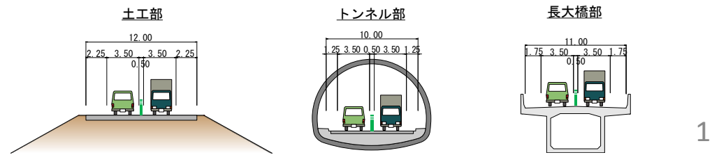
《標準横断図》
