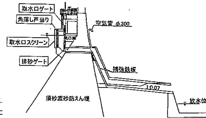
図-4 排砂路縦断面図(B-B)
