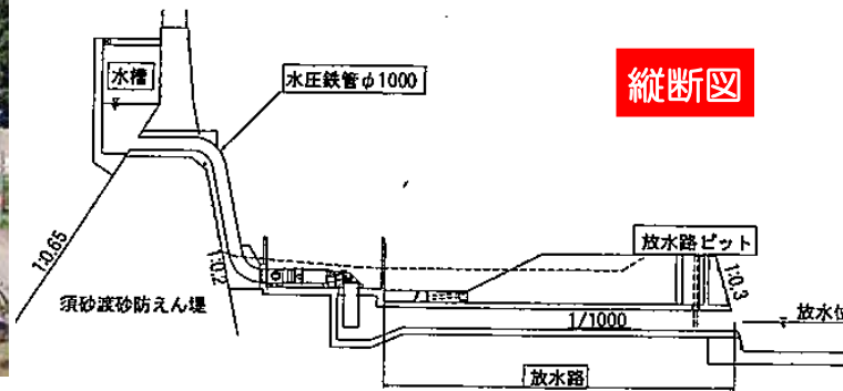
図-3 主水路縦断面図(A-A)
