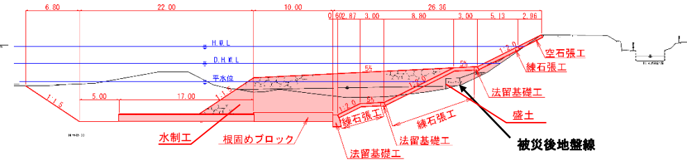
標準断面図(根固減勢部) B'-B
