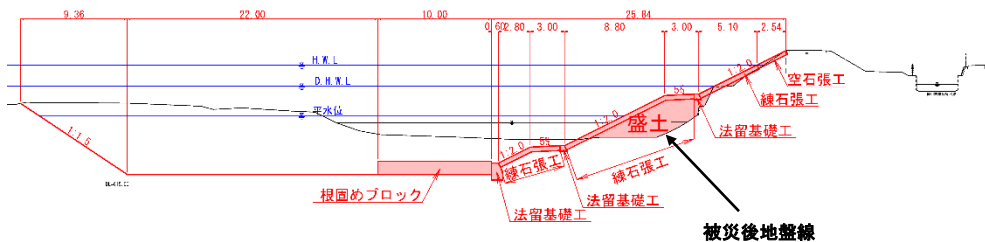
標準断面図(根固部) A'-A
