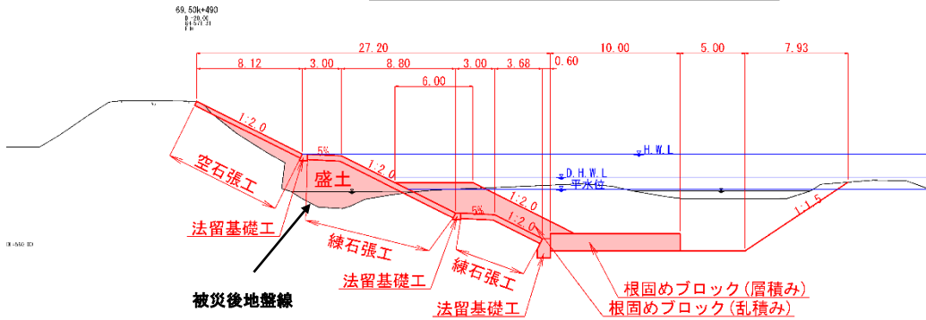
標準断面図 A'—A
